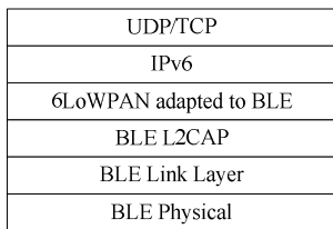
Figure 2. IPv6 over BLE Stack
